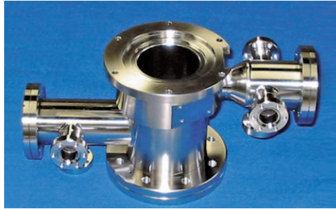
▲真空チャンバー (SUS,φ200)
