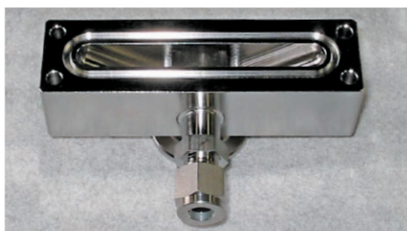
▲マニホールド (SUS, 200×70)
