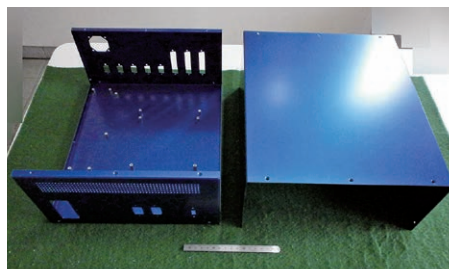
▲シャーシ (アルミ+青アルマイト)
