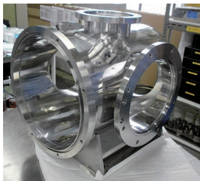
▲足付真空チャンバー (SUS)
