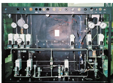
▲ガスパネル (700×300)
