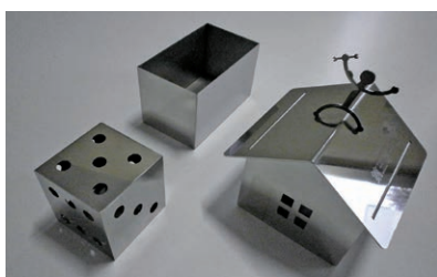
▲ファイバーレーザー溶接サンプル (SUS) ※左:t=0.8 上:t=0.5 右:t=1.0
