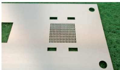
▲パターンプレート (インコネルt=0.5) ※写真中央、φ0.2、φ0.4、φ0.6
