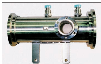
▲真空配管 (SUS, \phi 101.6 )
