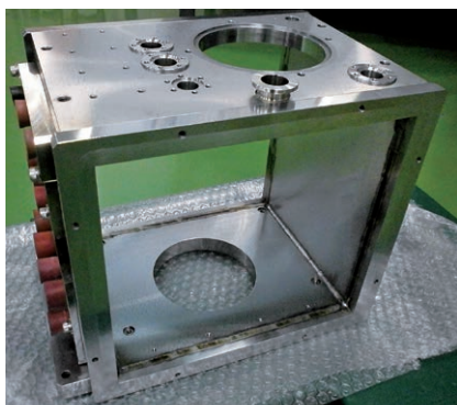
▲溶接角チャンバー (SUS)
