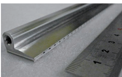
▲ブローノズル (拡大)
