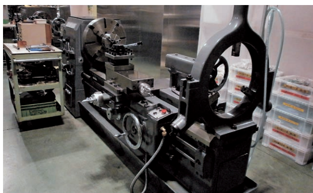
▲振れ止め付汎用旋盤
